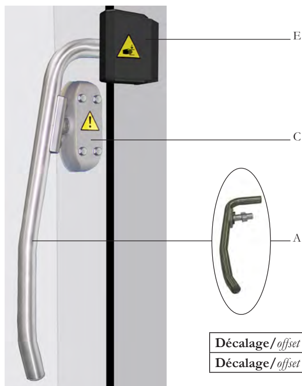
Poignée sans butée Handle without butt
