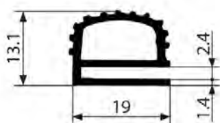
Bourrelet N°27
