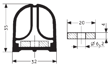
Bourrelet N°4450
