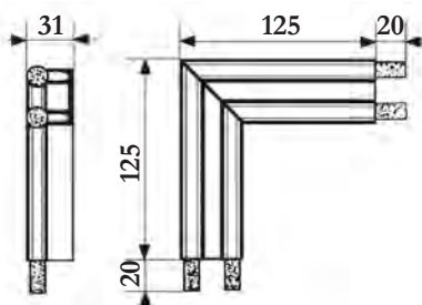
Pièce d'angle N°4453
