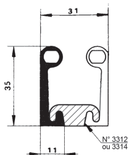
Bourrelet N°8511
