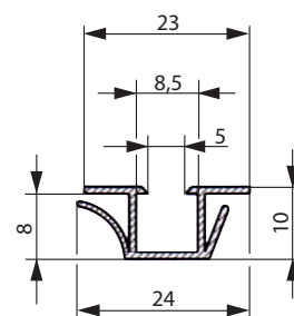
Raidisseur N°2962
