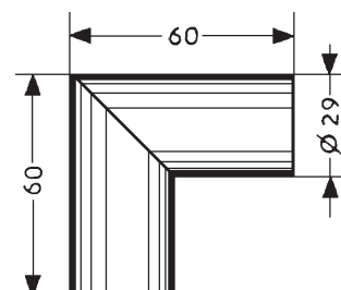
Pièce d'angle N°3462
