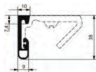
Bourrelet N°2350
