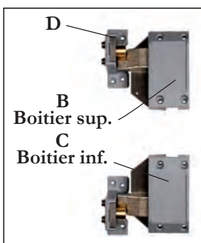
Points de serrage pour porte droite
