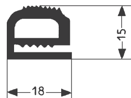
Bourrelet N°74
