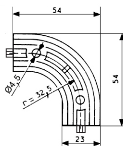
Raidisseur N°2313
