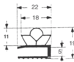
Bourrelet N°74
