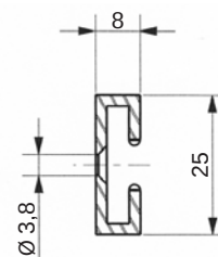
Raidisseur N°3352
