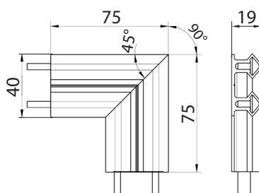
Angle pour bourrelet N°67
