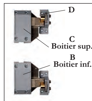
Points de serrage pour porte gauche
