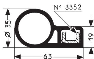
Bourrelet N°3461
