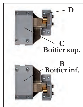
Points de serrage pour porte gauche
