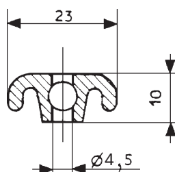
Raidisseur N°3362
