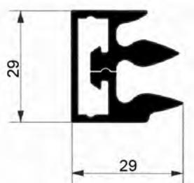
Raidisseur N°252
