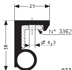
Bourrelet N°3350
