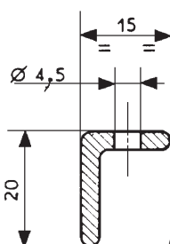
Raidisseur N°3362
