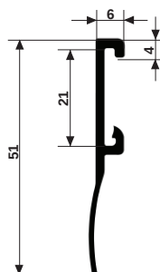
Raidisseur N°2313
